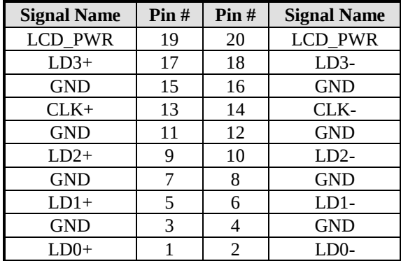
J18(Odd Bus),J19(Even Bus)
