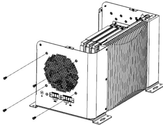
(Figure 4: Fan Removal)
